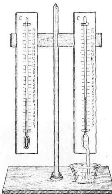
Рис. 12. Стационарный психрометр
